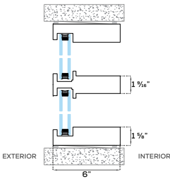
Transom Option
